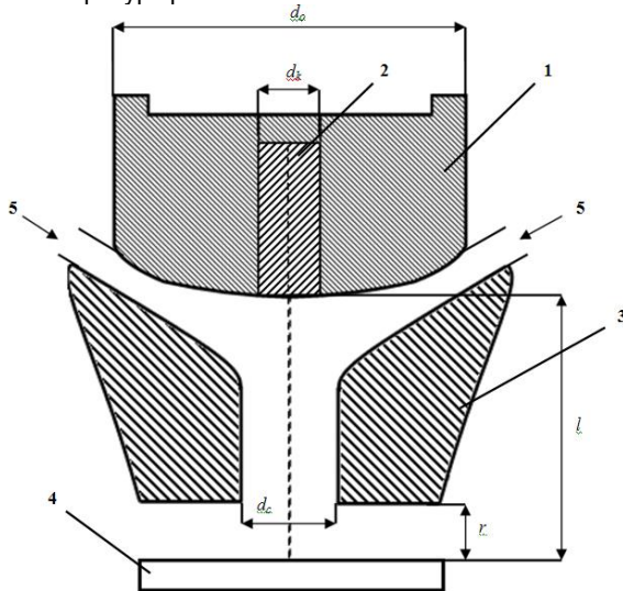
Рисунок 2. Схема плазмотрону прямої дії:
