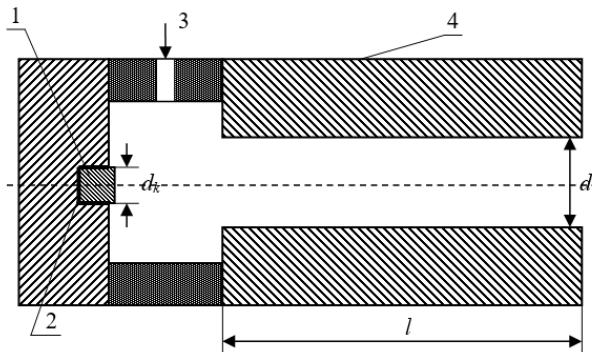
Рисунку 1. Схема плазмотрону: 1- катод, 2 - катодотримач, 3 - система подачі робочого газу, 4 - анод.
